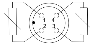
M12 Stecker 2x PT100 oder 2x PT1000
