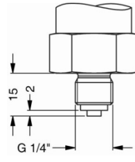
G1/4" EN 837
