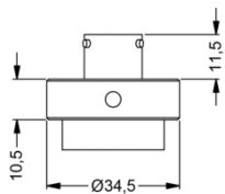
ISO 4400 (IP 65)
